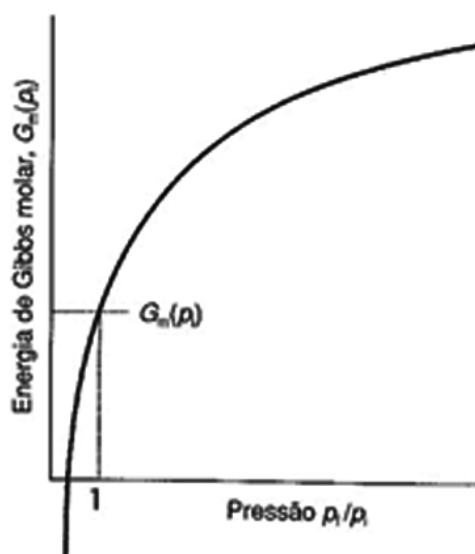
Figura 1.2: Variação da energia de Gibbs molar de um gás perfeito com a pressão.
