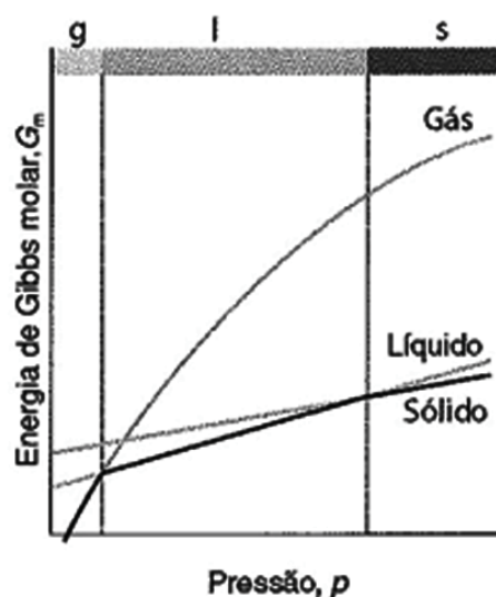
Figura 1.1: Variação da energia de Gibbs molar com a pressão.
