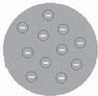
Modelo de Thomson
