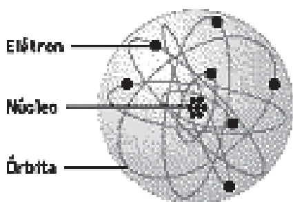
Modelo de Rutherford
