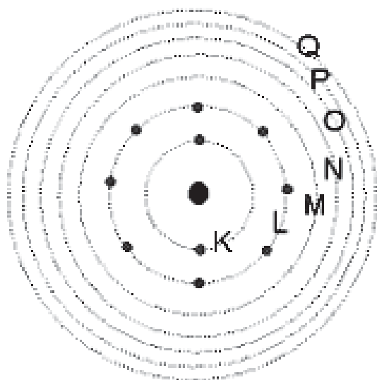
Modelo de Bohr.
