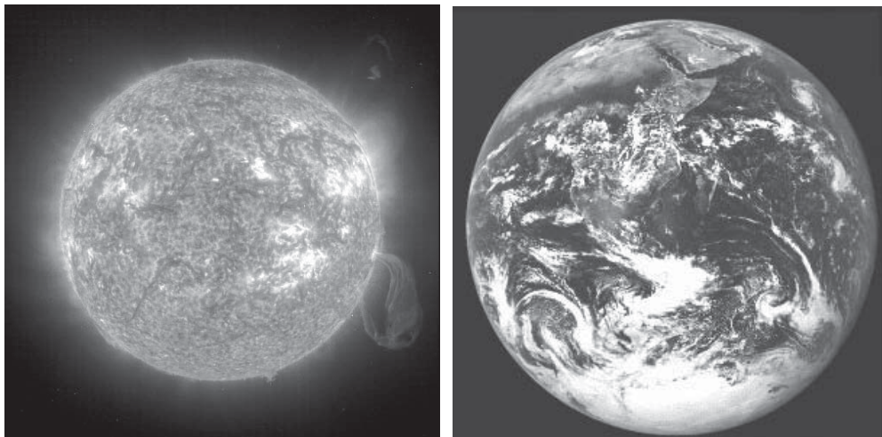
Sol; Terra (Fonte: http://www.astro.iag.usp.br ).
