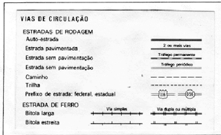
Figura 8: Vias de Circulação (Carta topográfica esc. 1:100.000).
