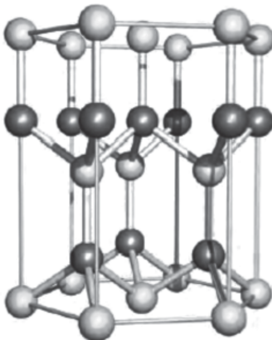
Figura 9: Representação da cela unitária em wurzita do ZnS ( Zn^{2+} : cinza; S^{2-} : amarelo) (Fonte: referência 6)
