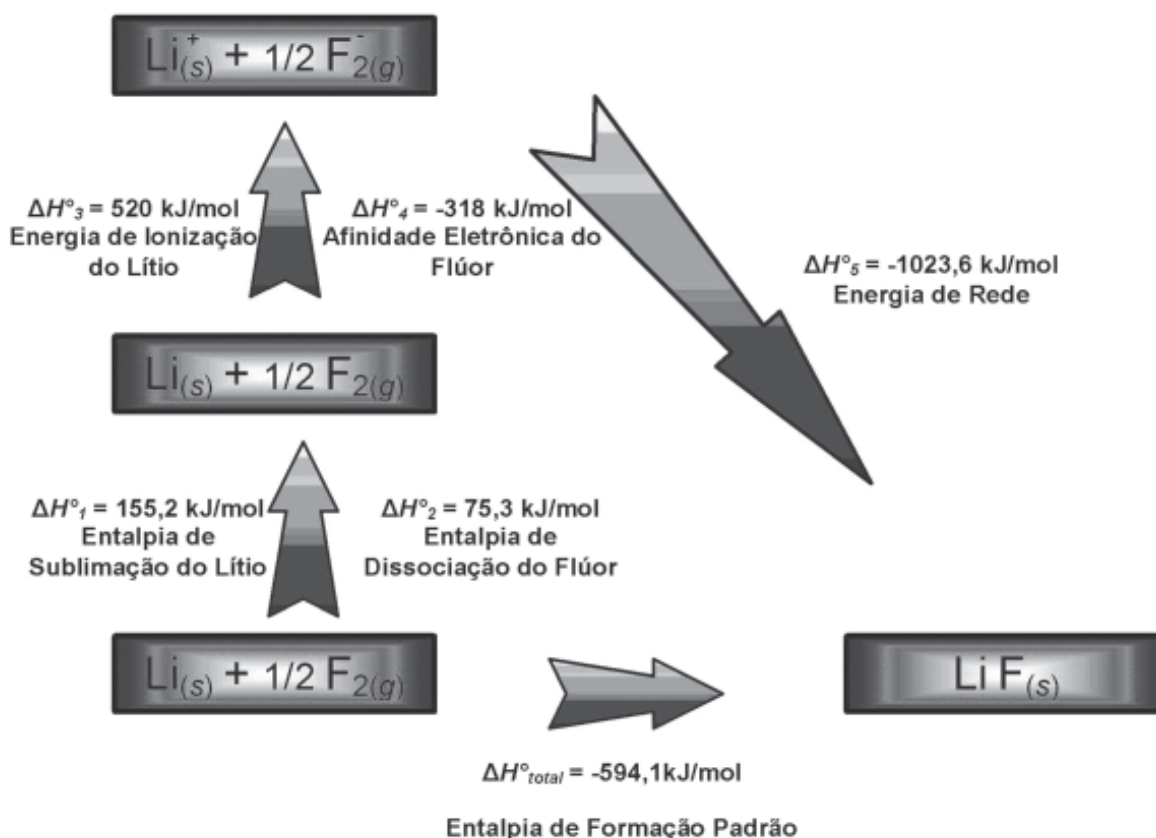
Figura 12: Ciclo de Born-Haber para formação do \text{LiF} .
