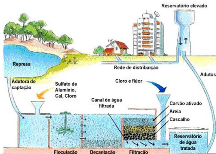
Representação esquemática de uma estação de tratamento de água. Fonte: http://www.cdcc.usp.br/ciencia/artigos/art_28/agua2.html Acessado em 03/01/2012
