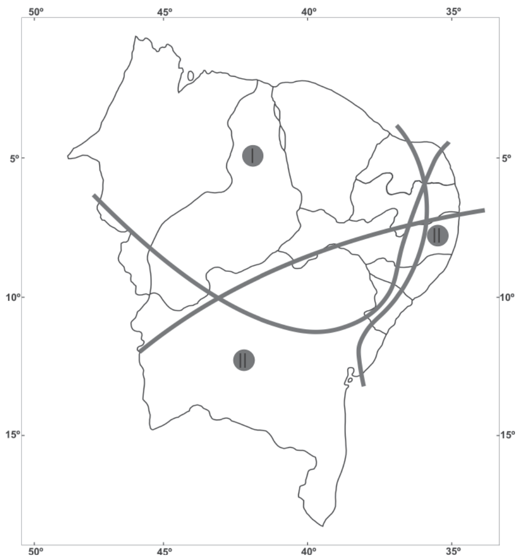
Fatores que influenciam a produção de precipitação pluvial no nordeste brasileiro.
