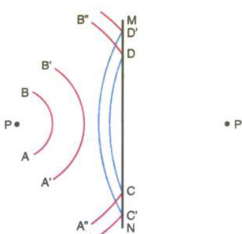
Figura 1 – Reflexão do Som
