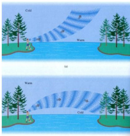
Figura 7 – Refração do Som. E. Hecht, Physics (Brooks Cole, 1994).
