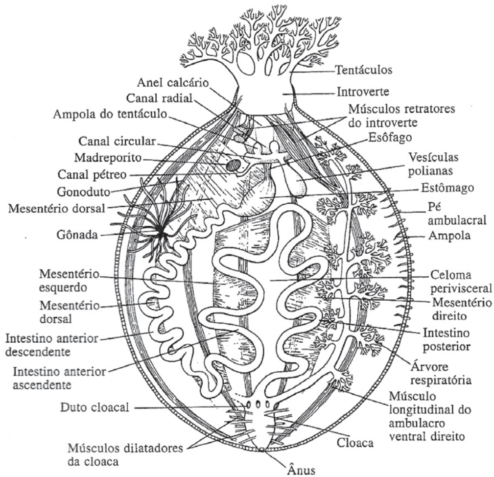
Anatomia interna de um holoturóideo mostrando todo sistema aquífero, muscular, respiratório, reprodutivo e digestivo
