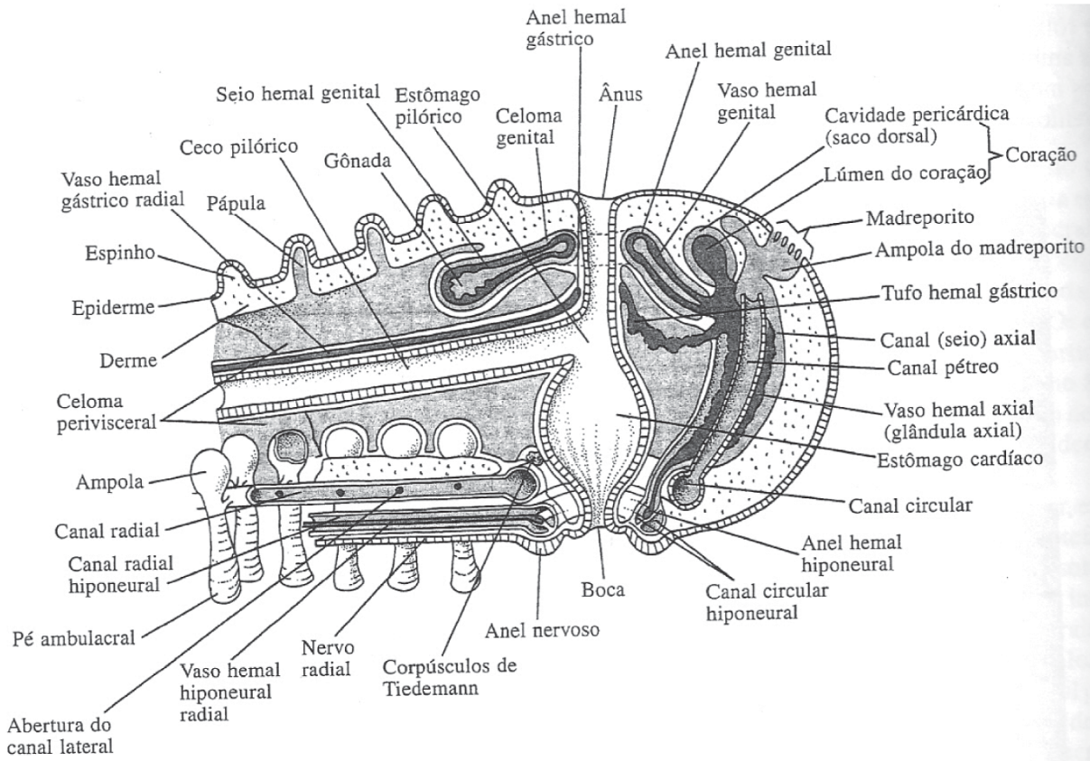
Corte da região central de uma estrela mostrando sistema digestivo e parte do ambulacrário
