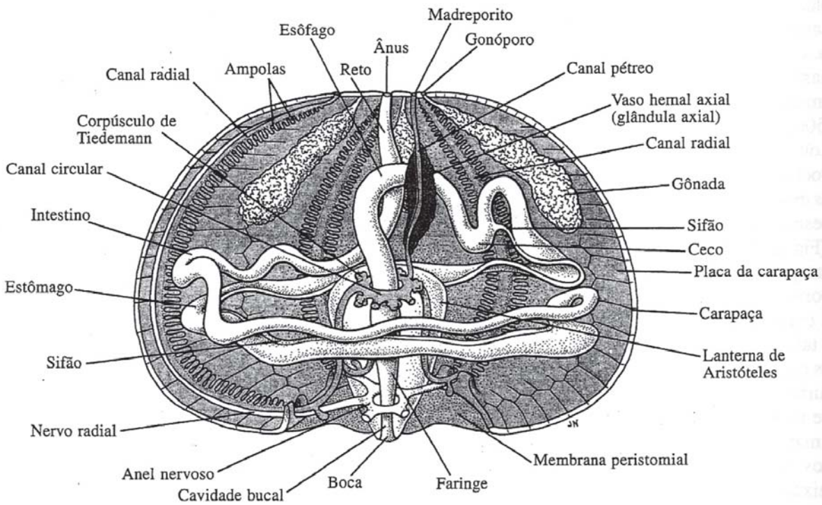
Anatomia interna de um equinóide (ouriço do mar) mostrando os sistemas aquífero, reprodutivo e digestivo
