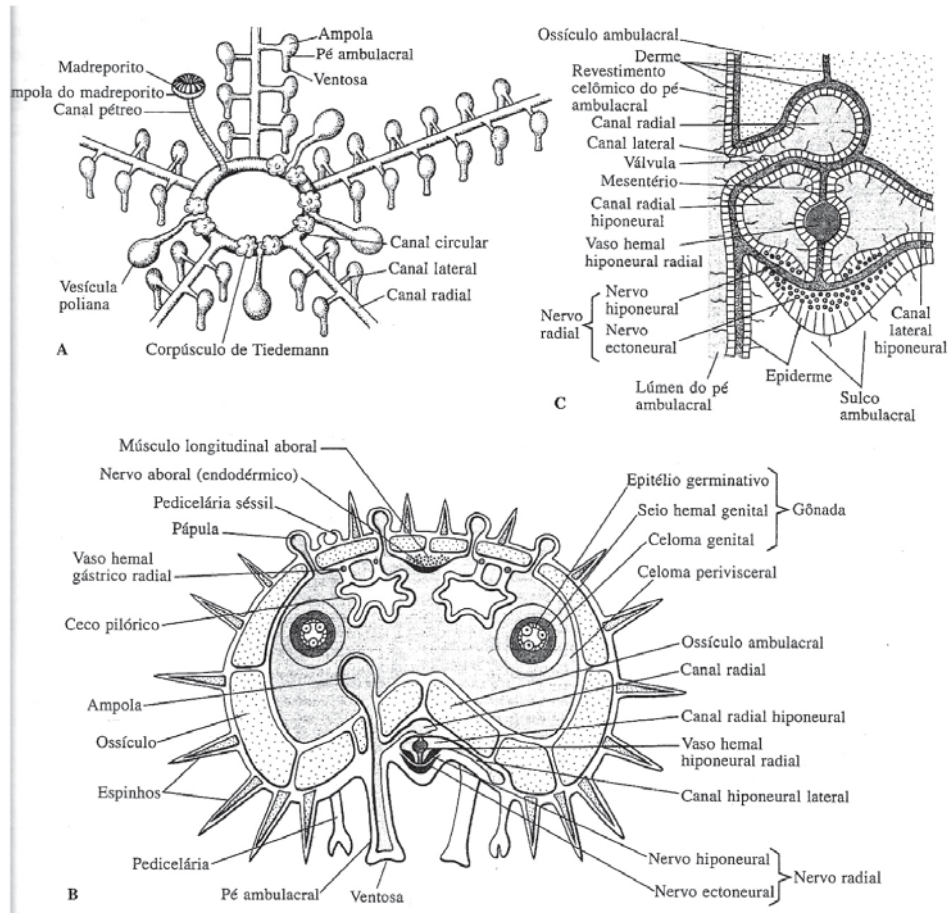
Esquemas do sistema ambulacrário de um equinodermo
