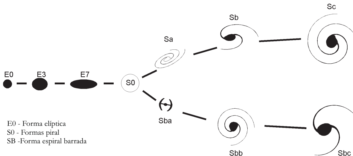
Figura 1.4 - Classificação morfológica das galáxias.
