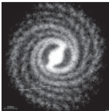
Figura 1.3 - Via Láctea (Fonte: http://www.adur-rj.org.br ).
