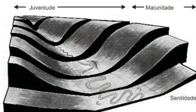
Figura 1.2 – Ciclo ideal com um relevo moderado. Fonte: Rice, 1992, In Cassetti, 1990.
