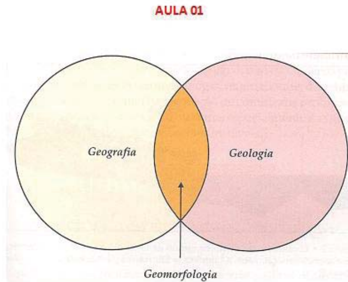
Figura 1.1 - A interseção da Geomorfologia com a Geografia e Geologia. Fonte: Jatobá e Lins, 2008.
