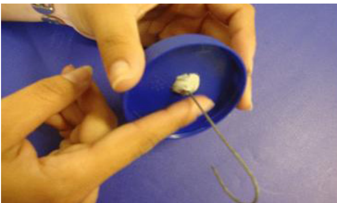
Fixação do arame na tampa com o adesivo epóxi.
