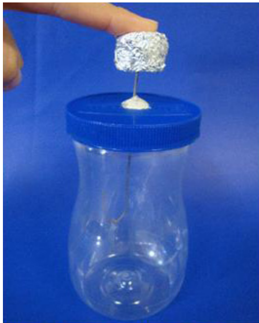
Processo realizado para fazer com que a esfera fique neutra novamente.
