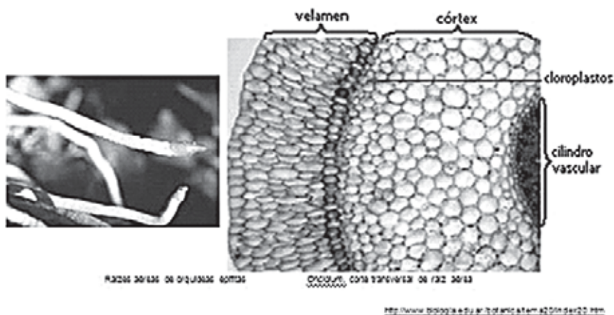
Figura 3 – Raízes aéreas de orquídeas epífitas (esquerda) e corte transversal de raiz aérea de Oncidium . (Fonte: http://www.biologia.edu.ar/botanica/tema20/index20.htm ).
