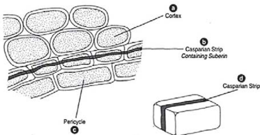
Figura 5 – A endoderme, uma única camada de células, possui as estrias de Caspary (b), que se localiza ao longo das paredes radiais e transversais. As estrias de Caspary são tidas como influentes sobre o fluxo de entrada/saída de água do córtex (a) para o periciclo (c) e vice-versa. (Fonte: Schooley). (1996).
