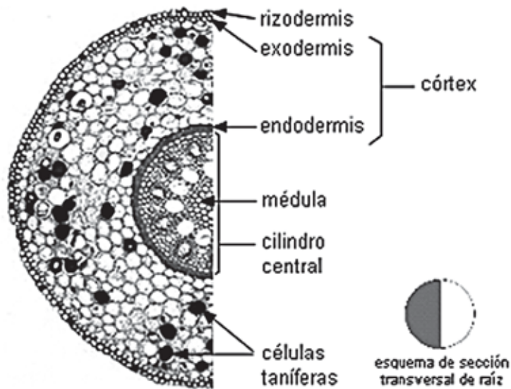
Figura 4 - Corte transversal mostrando as principais camadas da raiz. (Fonte: http://www.biologia.edu.ar/botanica/tema20/index20.htm ).
