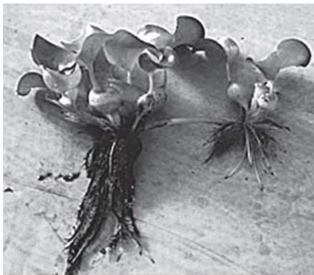
Figura 10 – Caules e raízes flutuantes de “aguapé”.
