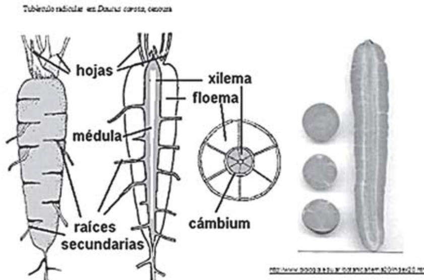
Figura 8 – Raiz tuberosa pivotante da cenoura ( Daucus carota ). (Fonte: http://www.biologia.edu.ar/botanica/tema20/index20.htm ).
