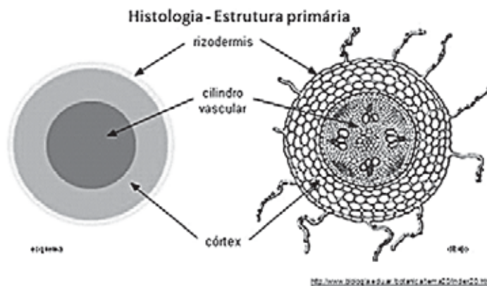
Figura 2 – Estrutura primária da raiz em corte transversal. (Fonte: http://www.biologia.edu.ar/botanica/tema20/index20.htm ).
