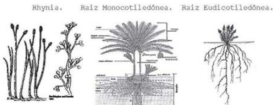
Figura 1 – Esquema estrutural de Rhynia † e do padrão de organização de raízes de monocotiledôneas e eudicotiledôneas. (Fonte: http://home.manhattan.edu/~frances.cardillo/plants/vascular/rhyniop.gif ).
