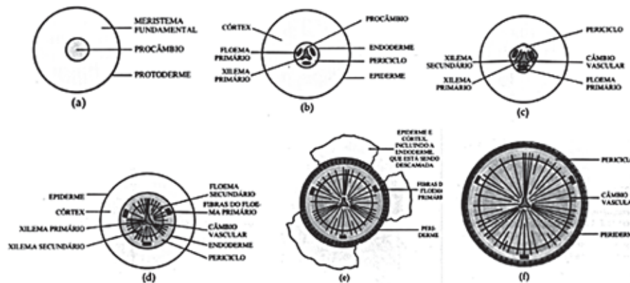
Figura 7 – Desenvolvimento da raiz de uma dicotiledônea lenhosa. (a) Em estágio inicial do desenvolvimento primário; mostrando meristemas primários. (b) Ao completar o crescimento primário, mostrando os tecidos primários mais o procâmbio entre o xilema e o floema primário. (c) Origem do câmbio vascular. Na raiz triarca, representada aqui, a atividade cambial se iniciou em três regiões independentes de procâmbio, entre os três cordões de floema primário e xilema primário. As células do periciclo opostas aos três pólos de protoxilema também contribuirão para formar o câmbio vascular recém-formado, de origem procambial. (d) Um pouco de floema e xilema secundários adicionais foram formados, separando posteriormente o floema primário do xilema primário. Uma periderme ainda não foi formada. (e) Em seguida, há a formação do floema e xilema secundários adicionais e de uma periderme. (f) No final do primeiro de desenvolvimento, mostrando o efeito do crescimento secundário – incluindo formação de periderme – no corpo primário da planta.
