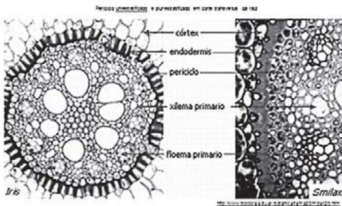
Figura 6 – Arranjo de sistema vascular em monocotiledôneas (Fonte: http://www.biologia.edu.ar/botanica/tema20/index20.htm ).
