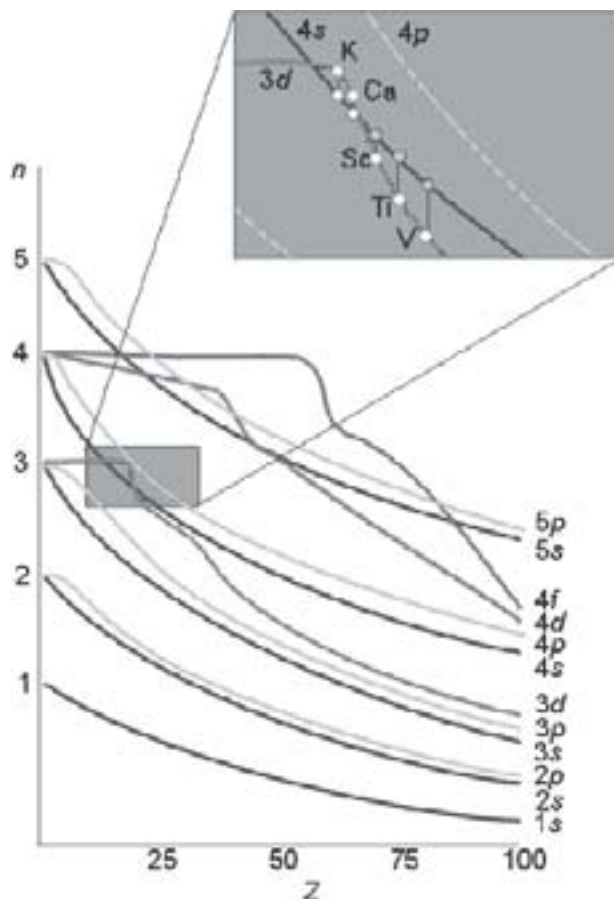
Figura 5: Uma representação mais detalhada dos níveis de energia de átomos multieletrônicos na tabela periódica. A inserção mostra uma vista ampliada próximo a Z=20 , onde os elementos 3d iniciam (Fonte: bibliografia 2).
