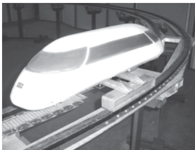
Figura 10: Protótipo de levitação magnética supercondutora, elaborada pelo Laboratório de Aplicação de Supercondutores (LASUP) da UFRJ ( www.dee.ufrj.br/lasup ).
