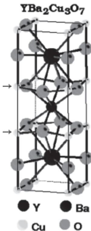
Figura 9: Estrutura do supercondutor YBa 2 Cu 3 O 7 ( www.searadaciencia.ufc.br ).
