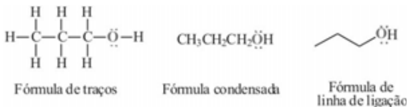
Figura 1: Representações estruturais para o álcool propílico
