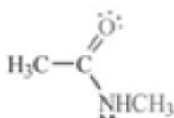
N-Metilacetamida
