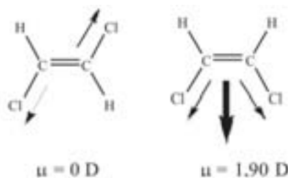
Figura 7: Momento de dipolo resultante do trans -1,2-dicloroetano
