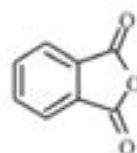
(Anidrido ftálico)
