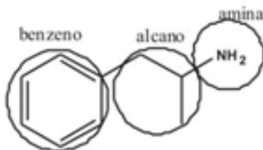
Anfetamina
